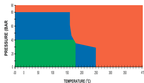
P- T DIAGRAM EN 1514-1, Type IBC, PN 40, DIN 28091-2/3.8, 2 mm
